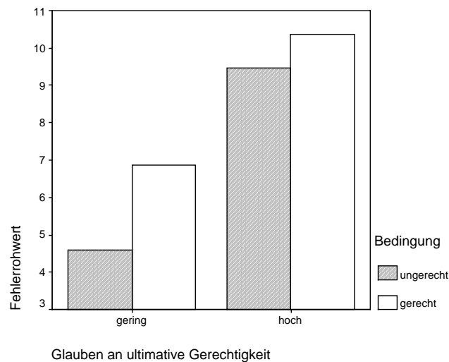
Abbildung 2: Grafische Darstellung der Mittelwertverteilung über die vier Zellen des Versuchsplanes auf der AV "Fehlerrohwert" im d2-Test
